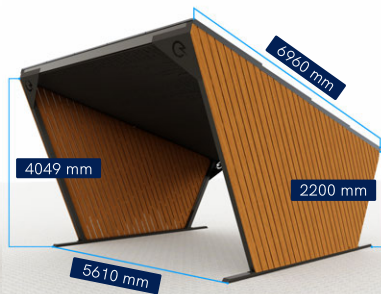
Solar Carport Modern Plus 7,8 kW
